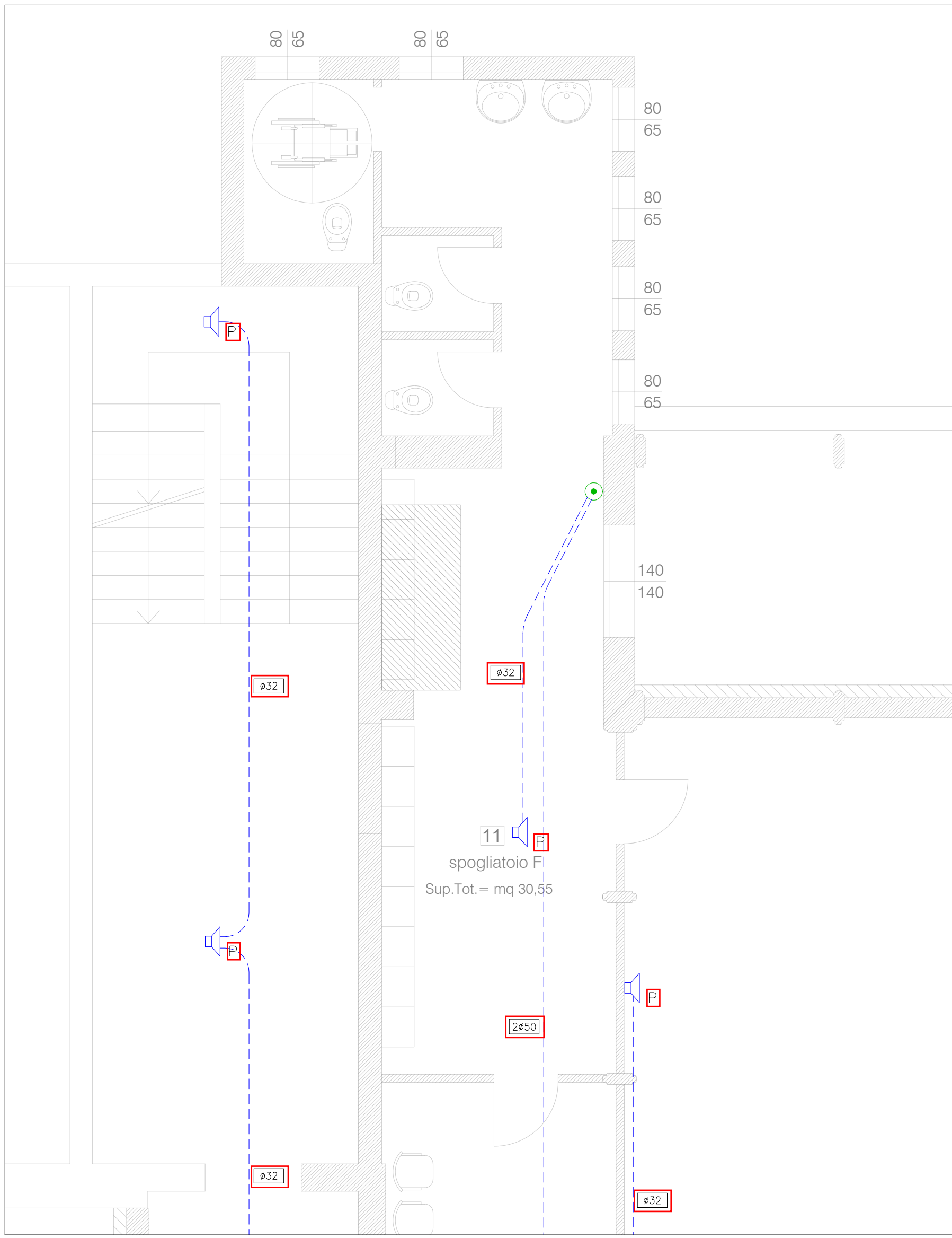
Planimetria piano secondo – Impianto EVAC spogliatoio F – Scala 1:50
